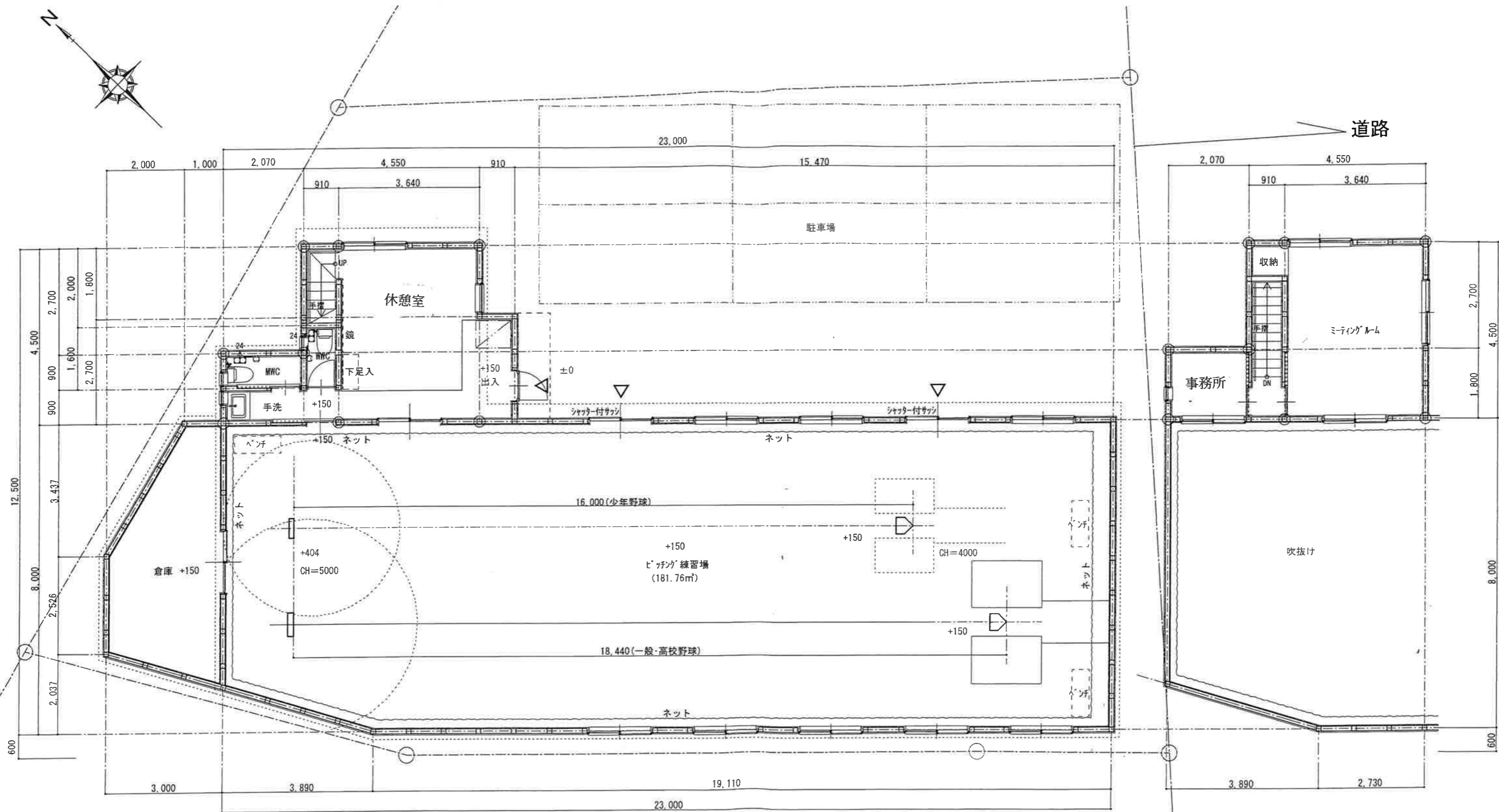
1階平面図 S=1:100 1階床面積 : 224.20㎡
